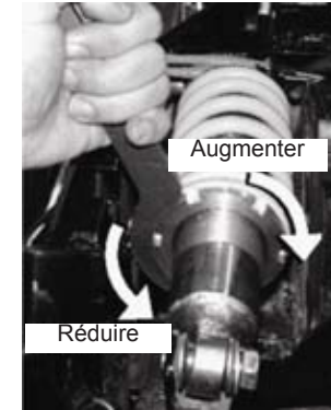
Figure 14 : réglage du ressort
